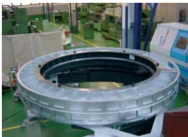
Rotador Nasmyth del GTC. © GRANTECAN
