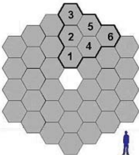
Grupo de segmentos que se someten a medidas "asociadas". © GRANTECAN
