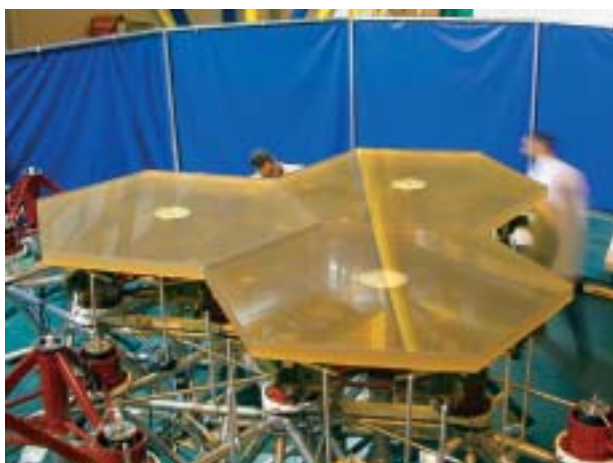
Segmentos montados en asociación con el segmento maestro para su pulido. © SAGEM
