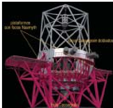
Estructura del GTC con los 7 focos. Autores: G. Pérez e I. Bonet (IAC)
